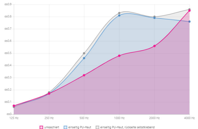
Schallabsorptionsgrad \alpha_s - Polyester Dichte 20kg/m 3 - t 20 mm
