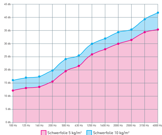
Schallabsorption in Anlehnung an ISO 140
